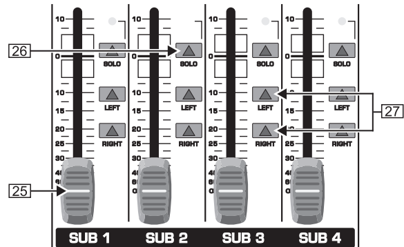
Fig. 2.9: Os subgrupos 1 - 4
