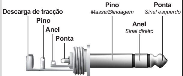
Fig. 5.6: Ficha jack estéreo para auscultadores
