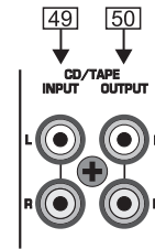
Fig. 2.21: Ligações CD/Tape
