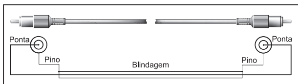
Fig. 5.3: Cabo Cinch
