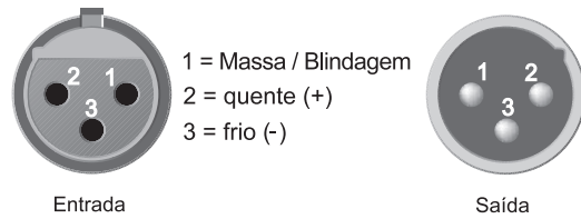
Fig. 5.4: Ligações XLR
